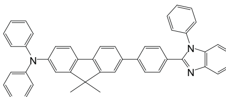
9,9-dimethyl-N,N-diphenyl-7-(4-(1-phenyl-1H-benzo[d]imidazol-2-yl)phenyl)-9H-fluoren-2-amine
