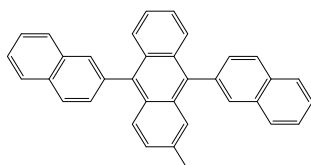
MADN
